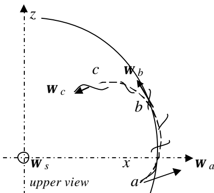
fig. 2.2 : Solar protuberance.
